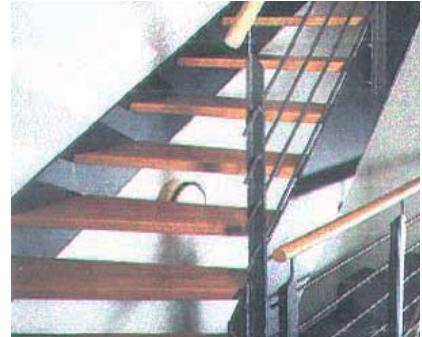
Stahlwangentreppe
