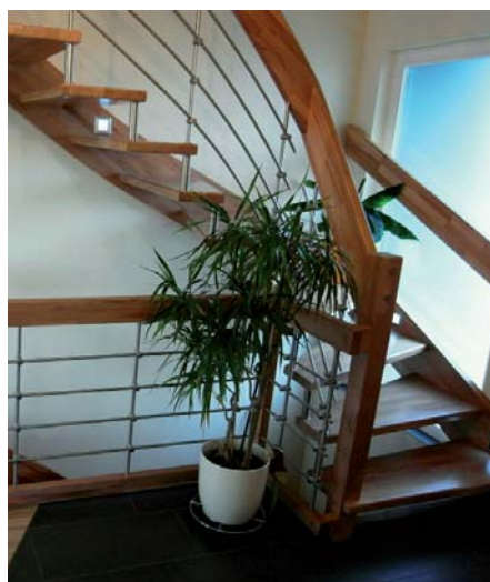
Bolzentreppe mit Wandwange
